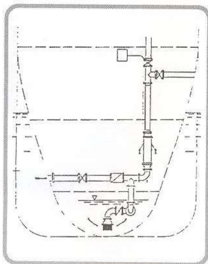
شکل ۷ - کنترل سطح آب در سیستم های ذخیره زیرزمینی
