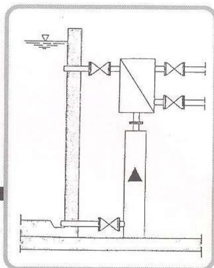
شکل ۹ - الف) مجموعه پمپ متصل به منبع
