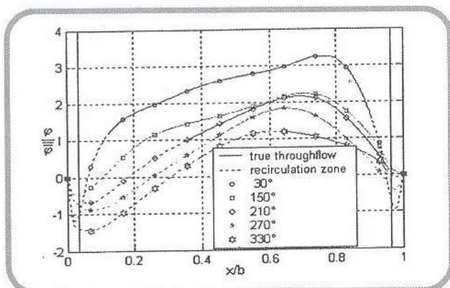
شکل شماره ۱۶ / \phi به ازاء موقعیت های محیطی مختلف \theta = 0.5\pi
