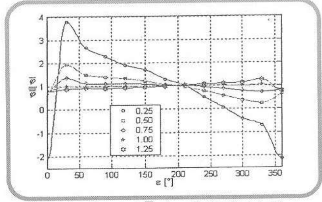
شکل شماره ۷ / مقادیر محلی \bar{Q} نسبت به موقعیت زاویه‌ای
