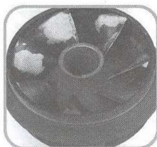
شکل ۱۰- a: پروانه‌های ساخته از CUSN۱۰-C پوشش onal۳۱۲zBel در اثر کایتاسیون پوسته پوسته شده‌اند b- جزئیات آسیب کایتاسیون
